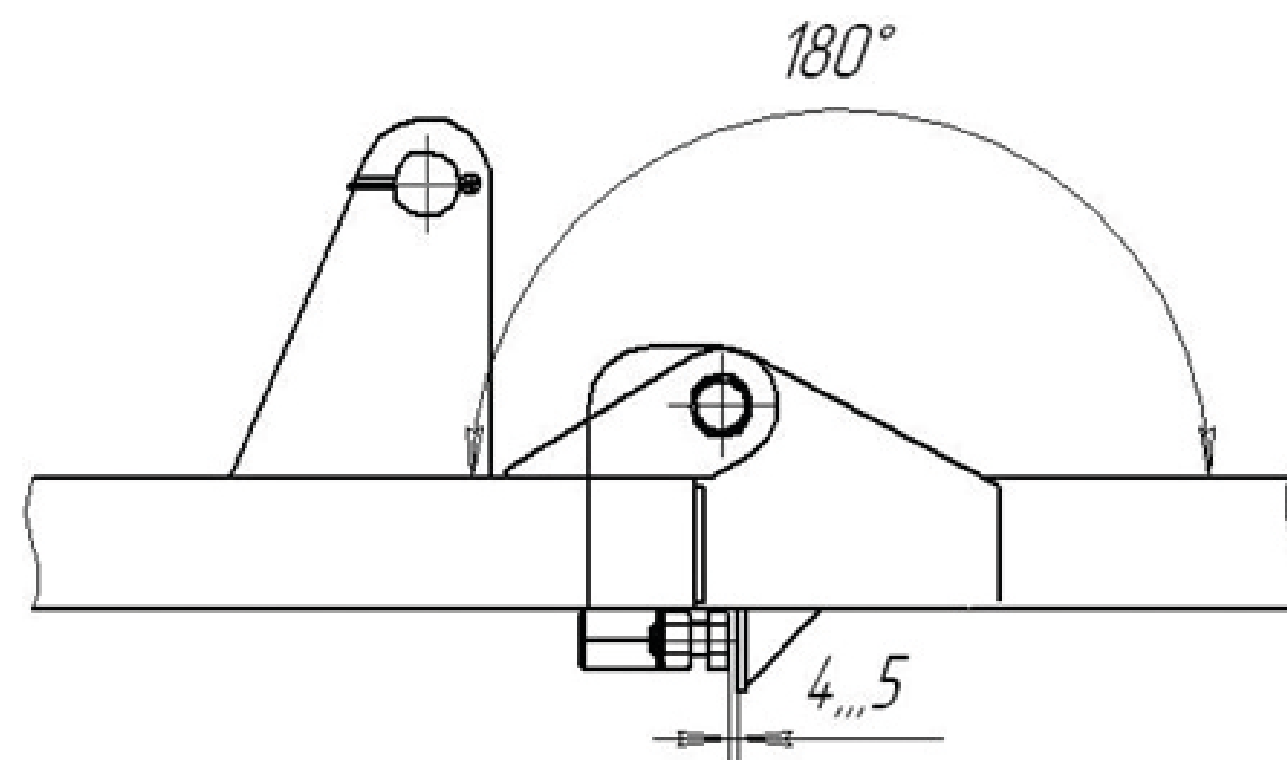
Рис. 10 Схема установки ограничительных винтов.
