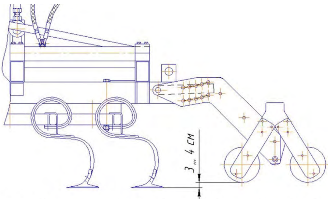
Рис.2а Предварительная регулировка рабочих органов культиватора KBM-ПД.
