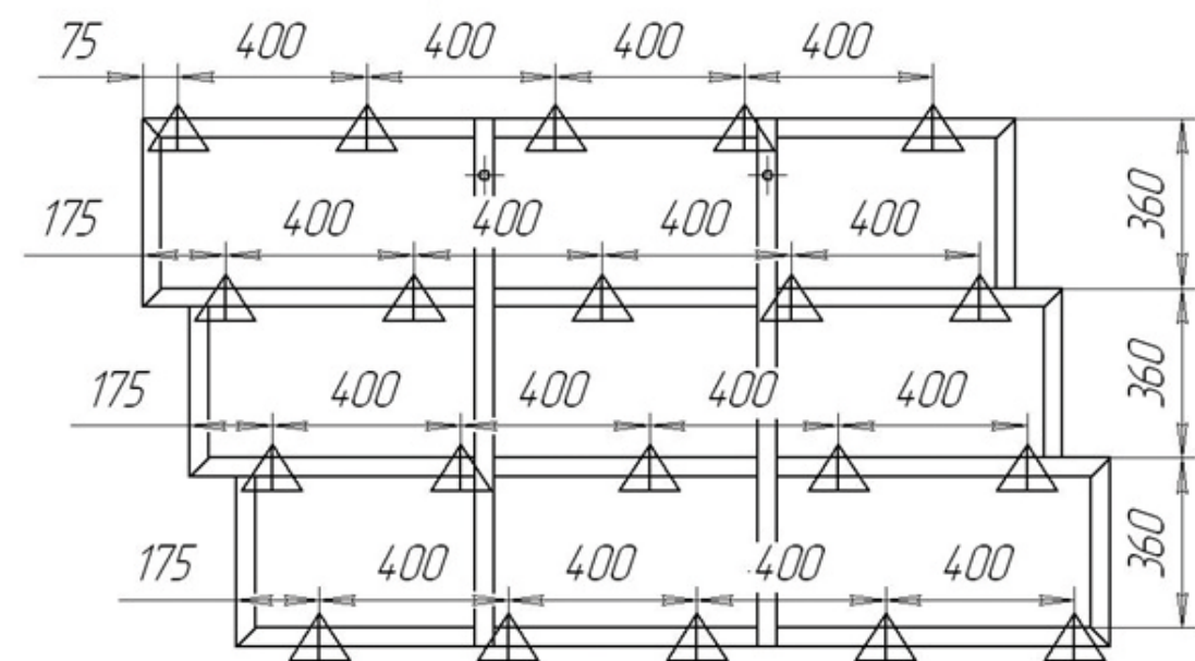
Схема расстановки рабочих органов КБМ-4,2; 6; 8.
