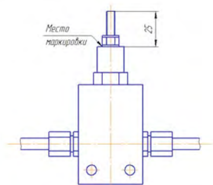
Рис.1 Предохранительный клапан.
