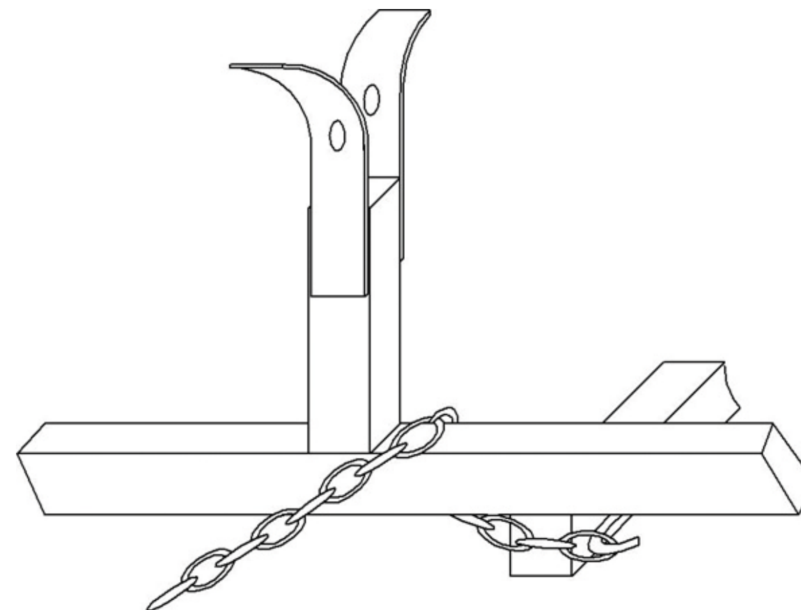
Рис. 3 Схема крепления натяжной цепи к боковой раме KBM-14,4 (15ПСВ).
