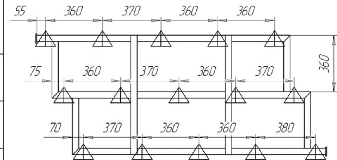
Схема расстановки рабочих органов КБМ-7,2; 10,8; 14,4.
