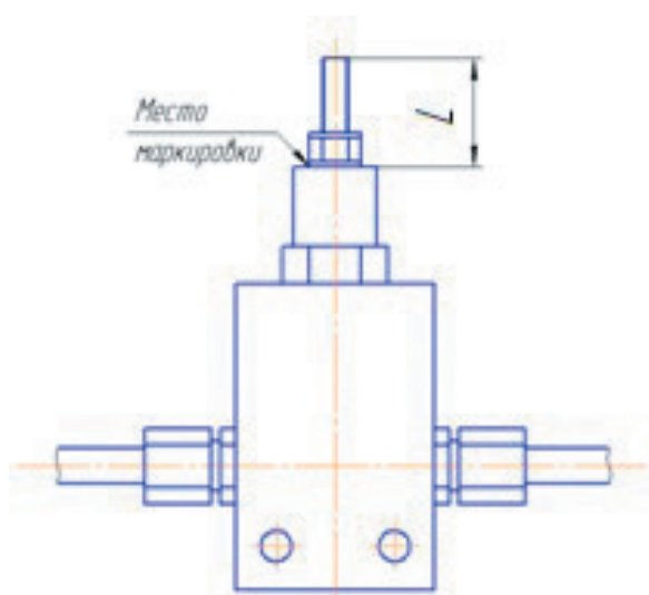
Рис.1 Приложения 2 Предохранительный клапан
