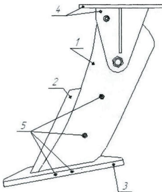
Рис. 2 Рабочий орган с кронштейном
